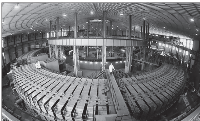
Синхрофазотрон
