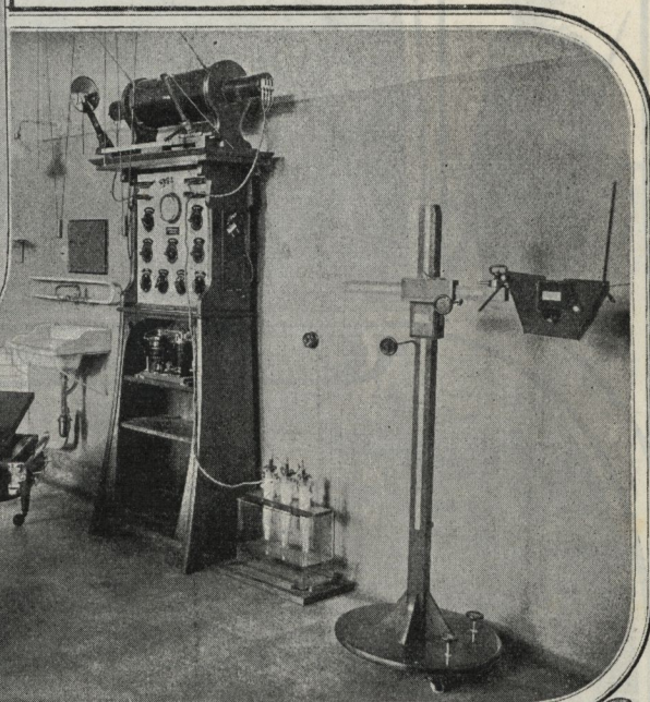
Рентгеновскій кабинетъ для изслѣдованія Рентгеновскими лучами. Большая Румкорфова спираль даетъ при разрядѣ искру въ 60 сантиметровъ длиною, могущую убить быка.
