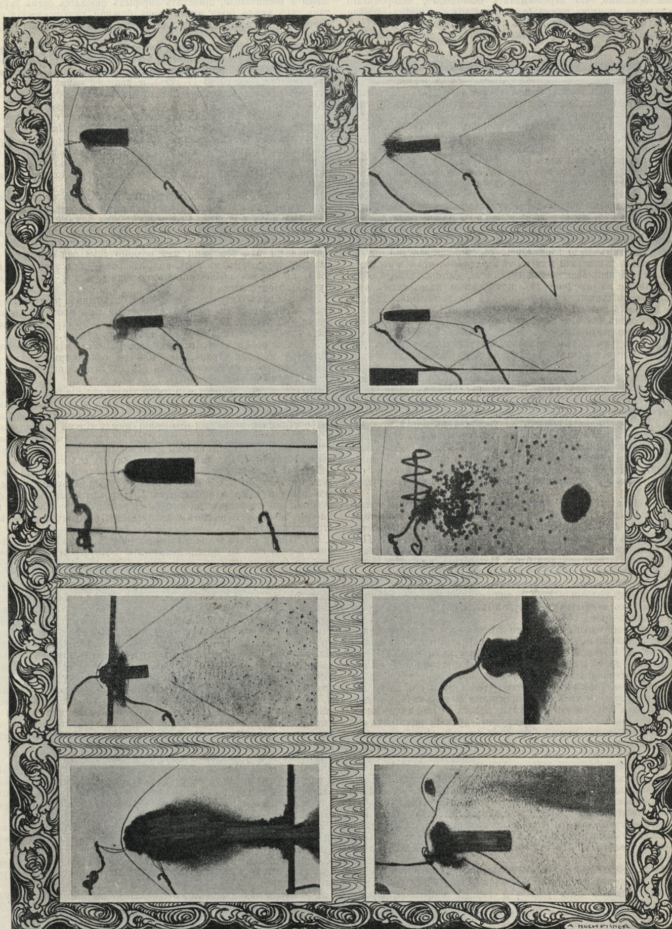
1 и 5. Пули системы Мартини-Генри, пролетающія 1.296 фут. въ секунду. 2. Пуля, летящая со скоростью 2.000 фут. въ секунду. 3. Пуля, летящая через пары эфира и карболовой кислоты. 4. Отраженіе отъ плоской поверхности воздушной волны, вызванной полетомъ пули. 6. Линіи воздушныхъ волнъ, вызываемыхъ полетомъ пули системы Шульца. 7. Пуля, пробивающая стеклянную пластинку и оставляющая за собою въ воздушныхъ волнахъ распыленные осколки стекла. 8 и 9. То же самое, но въ нѣсколько болѣе расплывчатомъ видѣ, при чемъ осколки стекла слились въ сплошную пыль. 10. Мелкія воздушныя волны, вызванныя разлетающимися во всѣ стороны осколками стекла.
